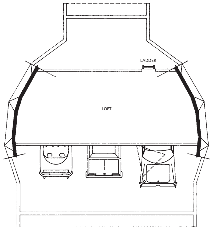
LOFT PLAN
